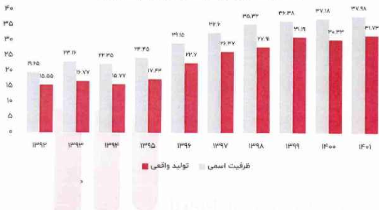
نمایه ۱۷: ظرفیت اسمی و واقعی آهن اسفنجی در ایران (ارقام به میلیون تن)
